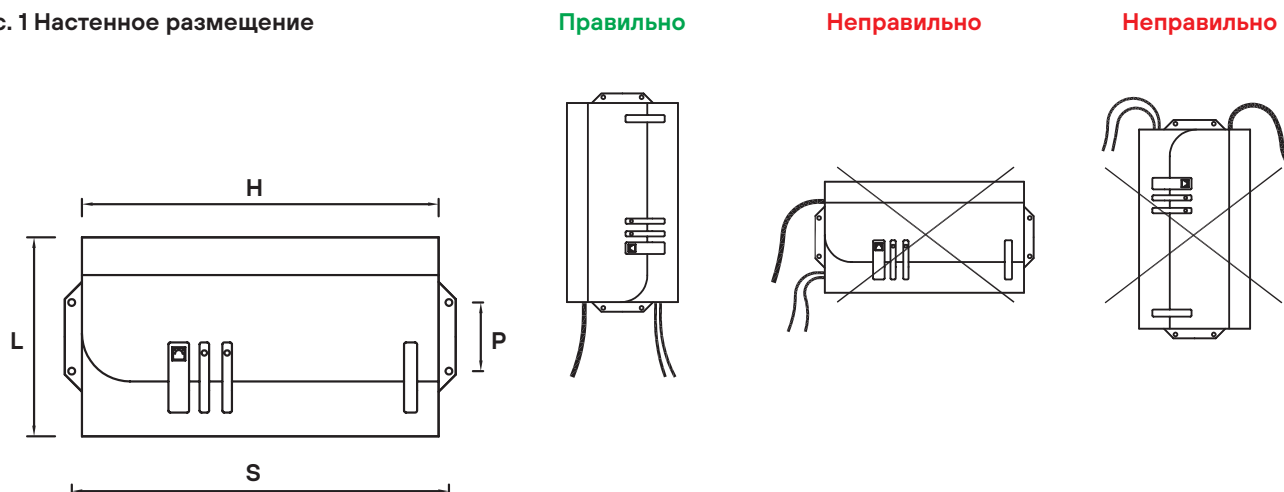
Рис. 2 Бортовое размещение
